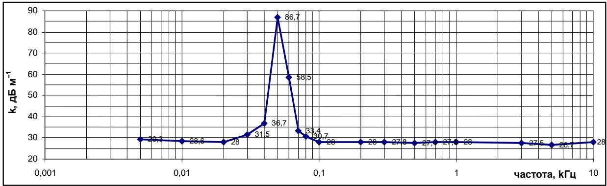
Рисунок 3 – Зависимость коэффициента калибровки k точечной магнитной антенны АИМ-НЧ.005.1 при внешнем магнитном поле \rho H = 131,5 дБ мкВ/м. Входное сопротивление измерителя 1 МОм
