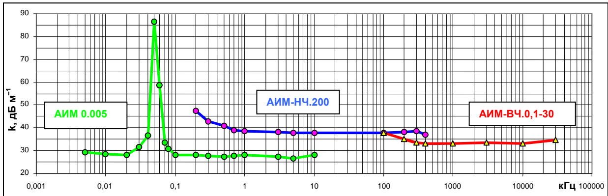
Рисунок 9 – Зависимость коэффициента калибровки точечных антенн АИМ 0,005 (с включенным режекторным фильтром 50 Гц); АИМ НЧ 200 и АИМ ВЧ 0,1-30 в частотном диапазоне 5 Гц ... 30 МГц.
