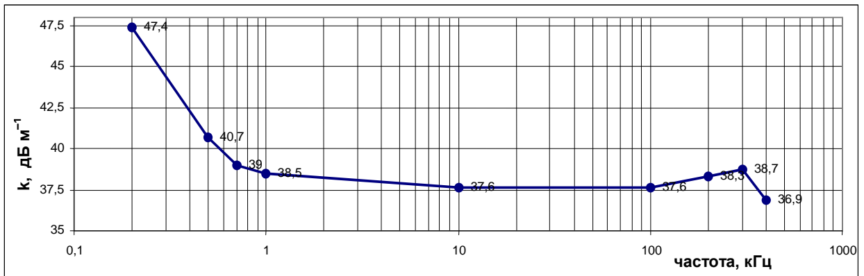
Рисунок 4 – Зависимость коэффициента калибровки k точечной магнитной антенны АИМ-НЧ.200.2 при внешнем магнитном поле \rho H = 131,5 дБ мкВ/м. Входное сопротивление измерителя 50 Ом.
