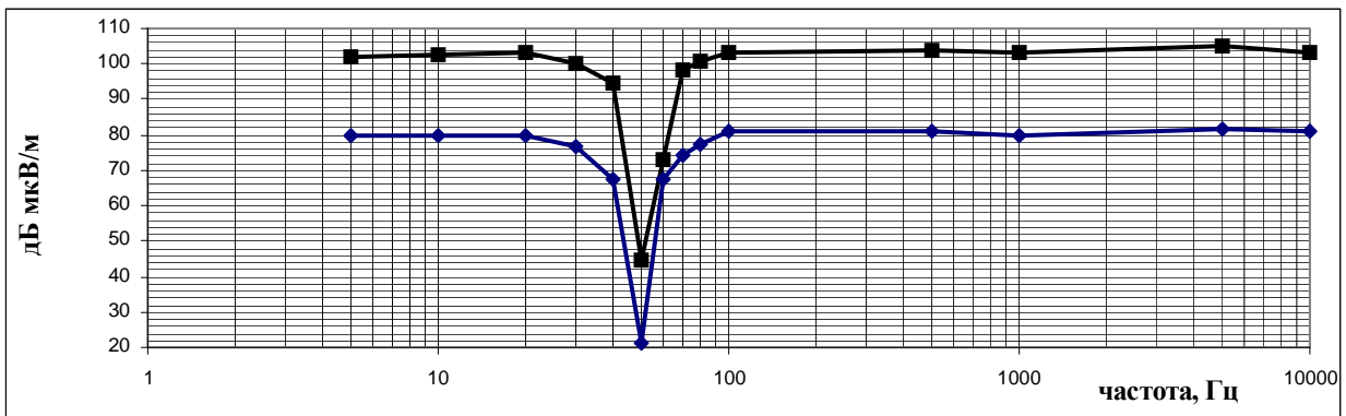
Рисунок 1 – АЧХ магнитной антенны АИМ-НЧ.005.1 при внешнем магнитном поле рН = 131,5 дБ мкВ/м. Верхняя кривая соответствует измерителю с входным сопротивлением 1МОм (UNIPAN237 с фильтром 40 дБ/окт), нижняя – измерителю с входным сопротивлением 50 Ом
