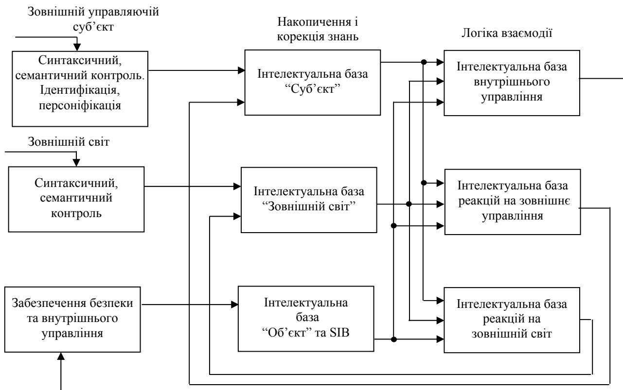
Рисунок 6 – Узагальнена функціональна (логічна) структура інтелектуального управління та забезпечення безпеки
