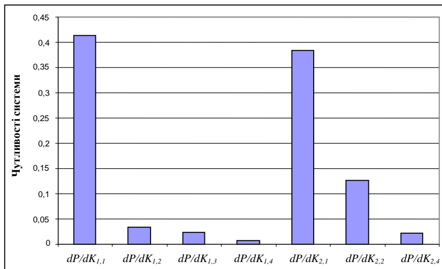
Рисунок 1 – чутливості системи захисту до зміни коефіцієнтів міцності
