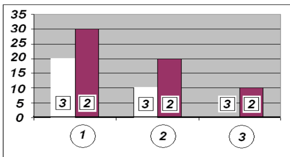
Рисунок 8 — Рівні гармонік, виміряних в точках 1, 2 і 3, згідно з рис. 3 при А= мінус 10 дБ, В= мінус 30 дБ
