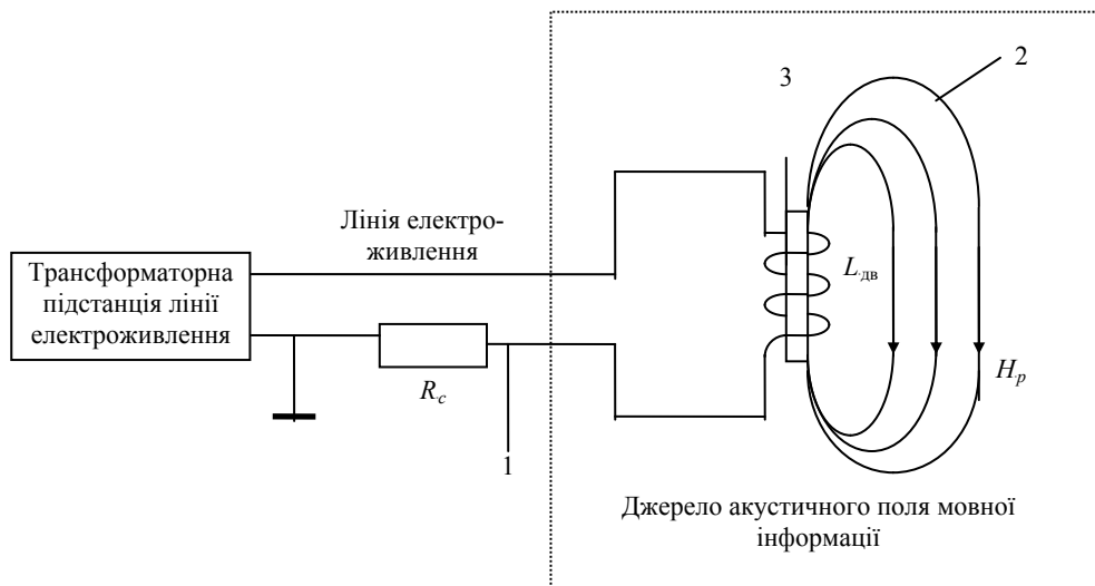
Рисунок 1– Виникнення віброакустичних кондуктивних і просторових каналів витоку мовної інформації (1 – віброакустичний кондуктивний канал витоку інформації; 2 – просторовий віброакустичний канал витоку інформації; 3 – магнітне осердя; R_c – сигнальний резистор; L_{дв} – індуктивність обмотки двигуна)
