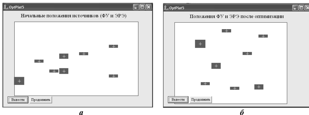
Рисунок 4 – Размещение ТВЭ на плате при оптимизации температур a – до оптимизации; б – после нее
