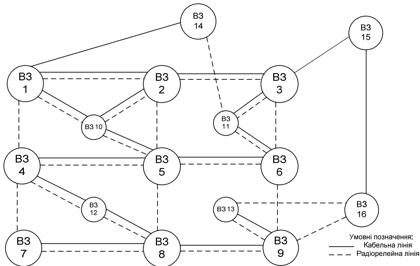
Рисунок 1 – Варіант побудови опорної мережі зв'язку
