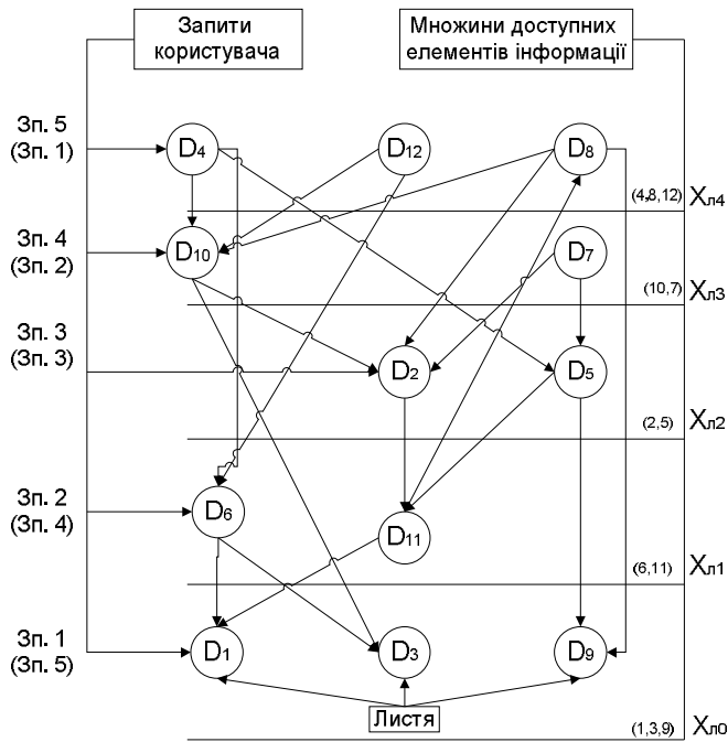
Рисунок 9 – Орграф структури інформаційних ресурсів із врахуванням вимог захисту (лісоподібна структура із закріпленими коренями / видалено дуги \langle D_{11}, D_8 \rangle ).
