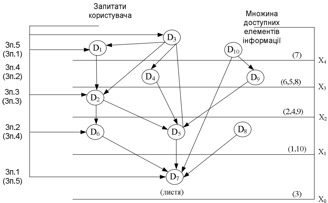
Рисунок 2 – Лісоподібна конфігурація структури інформаційного ресурсу (орграф із залежними листями)
