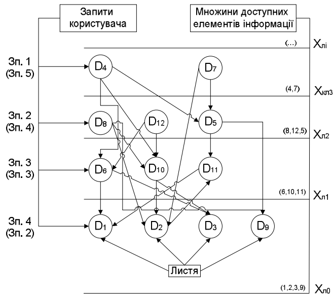
Рисунок 11 – Орграф структури інформаційних ресурсів із врахуванням вимог захисту (лісоподібна структура із закріпленими коренями / видалено дуги \langle D_2, D_{11} \rangle , \langle D_{11}, D_8 \rangle )
