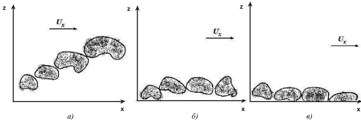
Рисунок 1 – Поширення хмари аварійно хімічно небезпечної речовини в атмосфері: а) - легкий газ; б) – газ, густина якого рівна густині повітря; в) - важкий газ
