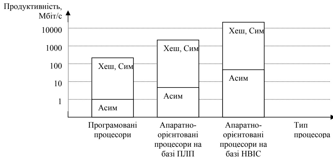
Рисунок 1 – Досягнуті рівні продуктивності виконання криптографічних алгоритмів на процесорах різної архітектури: Хеш – хеш-функції, Сим – симетричні шифри, Асим – асиметричні шифри, ПЛП – програмований логічний пристрій, НВІС – надвелика інтегральна схема.
