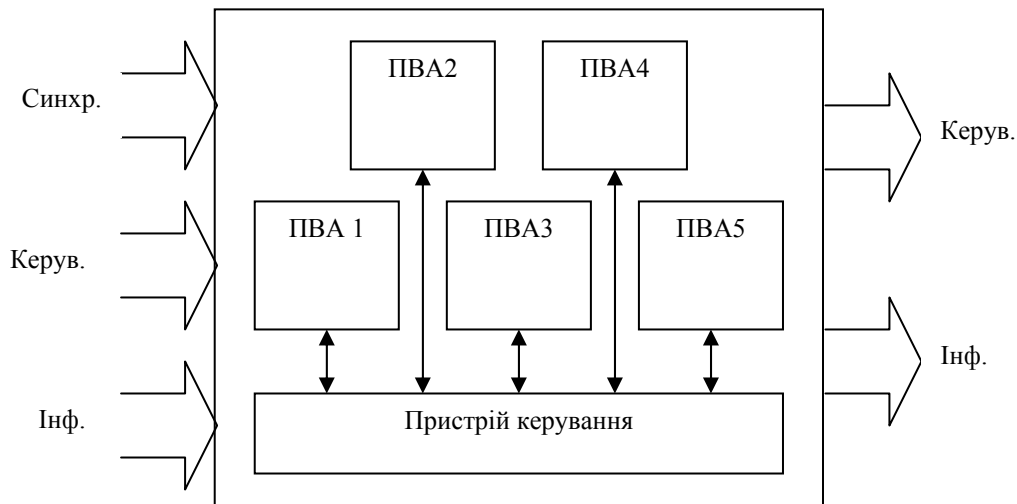
Рисунок 2 – Структурна схема процесорів виконання криптографічних функцій: ПВА – пристрій виконання алгоритму.
