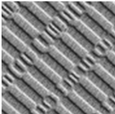
Рисунок 2 – Магнитный рельеф поверхности жесткого диска, полученный с помощью MFM
